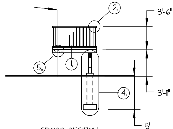
CROSS SECTION Scale: 1/8" = 1' - 0"
